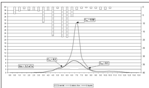
Fig.8: Sedimentogramma simulato della colata detritica in Val della Vecchia.
